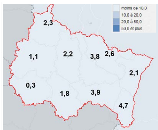
Figure 1 : Taux d'incidence pour Covid-19 sur 7 jours glissants par département de domicile en région Grand Est à la date du 5 juillet 2020. (Source: Laboratoires de ville et hospitaliers effectuant les analyses Sars-Cov-2)
